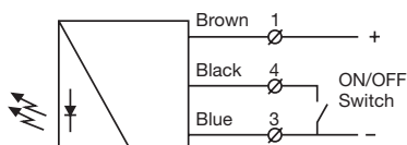
SPT 2645
