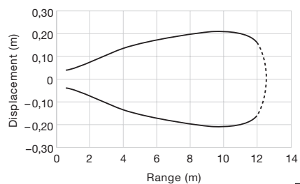
SPRR 2x12
