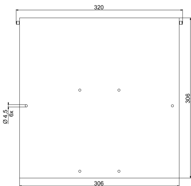
Vorderansicht mit Smart Shelf-Antenne
